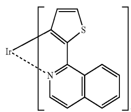
Ir(tiq) 3
