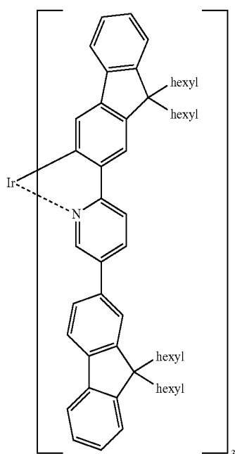
Ir(HFP) 3
