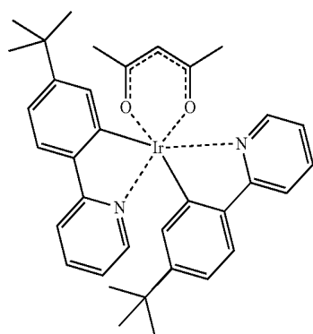
Ir(t-Buppy) 2 (acac)
