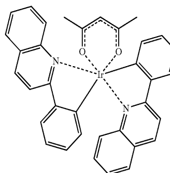
Ir(pq) 2 (acac)
