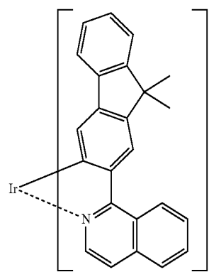
Ir(fli1) 3
