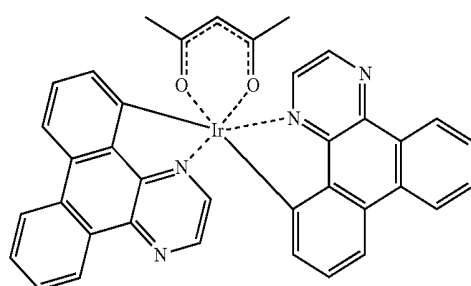
Ir(DBQ) 2 (acac)
