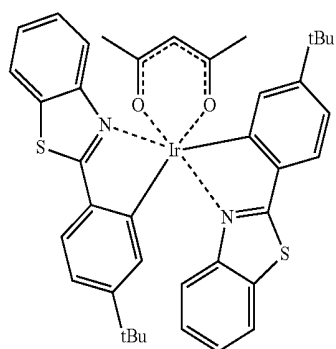
(t-bt) 2 Ir(III)(acac)
