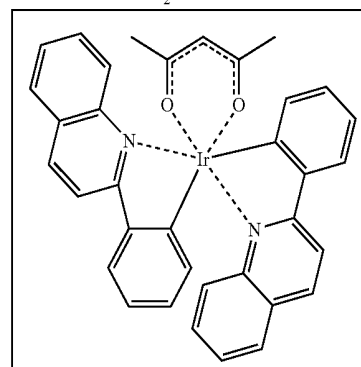
Ir(piq) 2 (acac)
