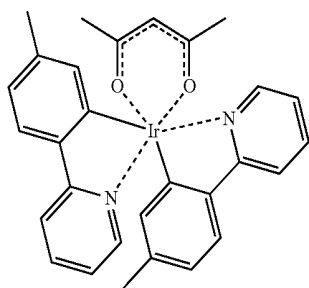
Ir(mppy) 2 (acac)
