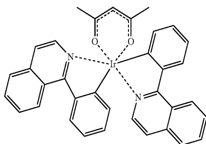
Ir(piq) 2 (acac)
