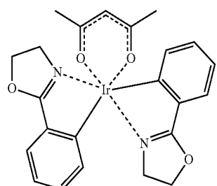
Ir(op) 2 (acac)
